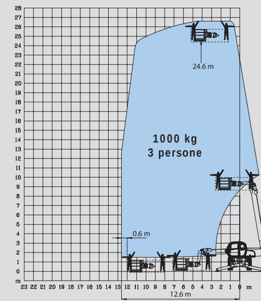
ROTAZIONE SU STABILIZZATORI COMPLETAMENTE SFILATI CON CESTELLO AERIAL JIB 2
